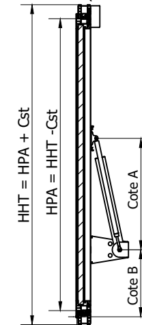
B-B ( 1:15 )
